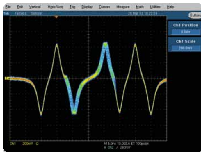
► Figure 27. Region shift.
